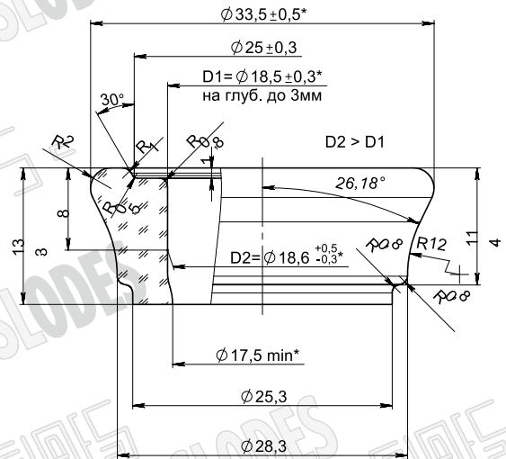
Венчик типа П-34 МАСШТАБ 3:1
