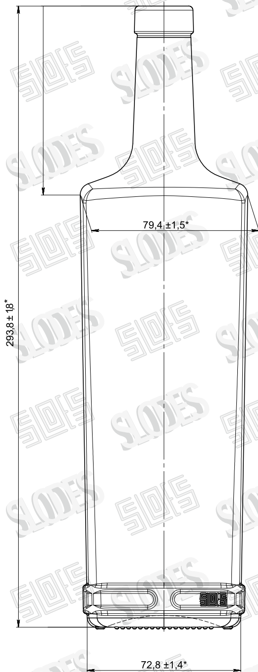
ВИД СПЕРЕДИ
