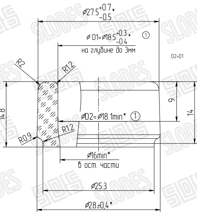
ВЕНЧИК (3:1)
